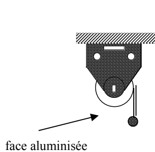
Montage plafond (1)
